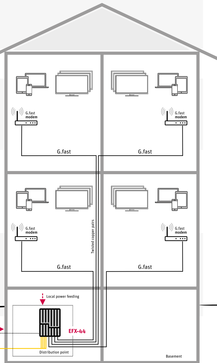
FTTB example
